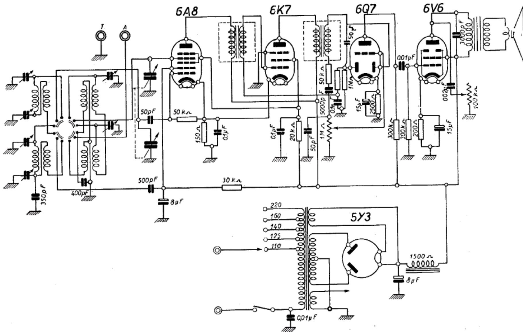
VARA RADIO - Mod. 509 S - Gamma medie da 200 a 600 m, gamma corte da 16 a 52 m. Media frequenza 467 kc/s. Potenza d'uscita 3 W. Consumo 50 W.
